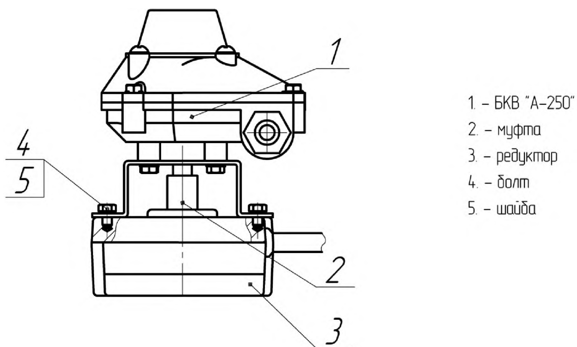
Рис. 5. Редуктор с БКВ «А-250».
