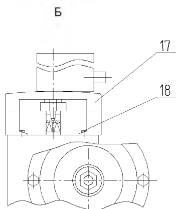
Рис. 7а. Пневмогидропривод с БКВ «Festo» и пневмораспределителем.
