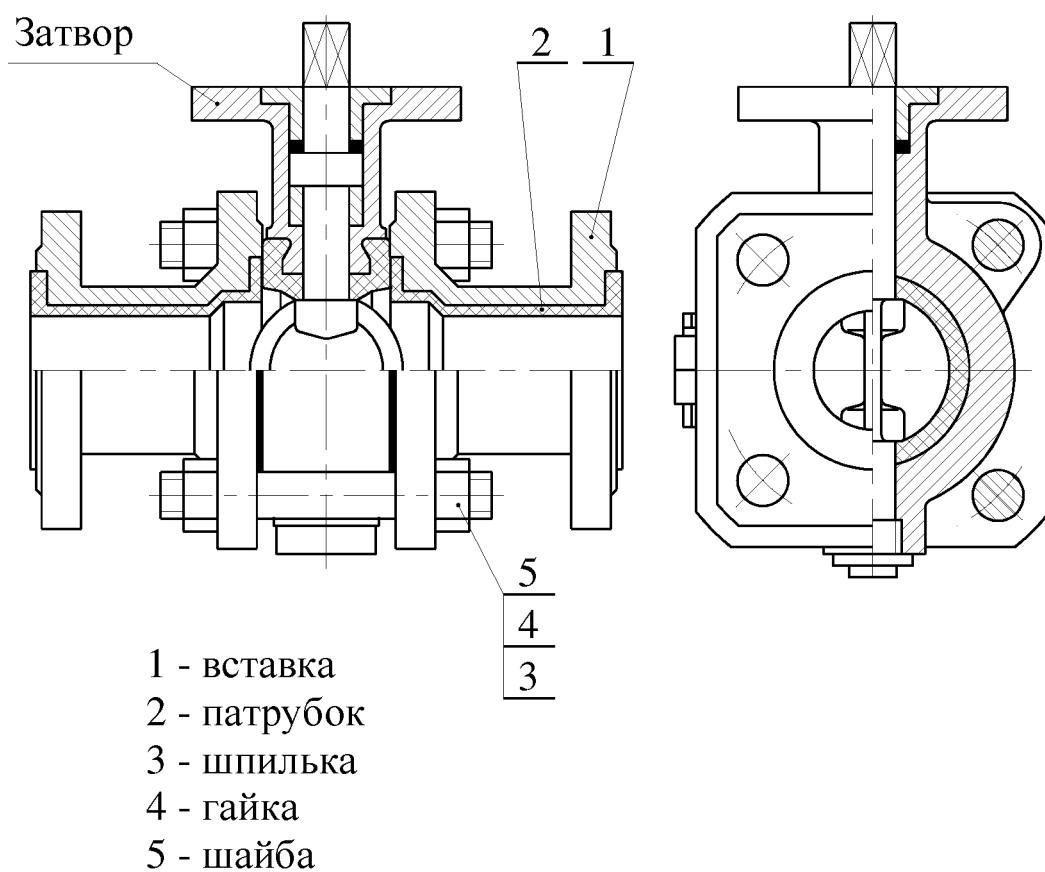
Рис. 12. Затвор DN 32-40 без органов управления.
