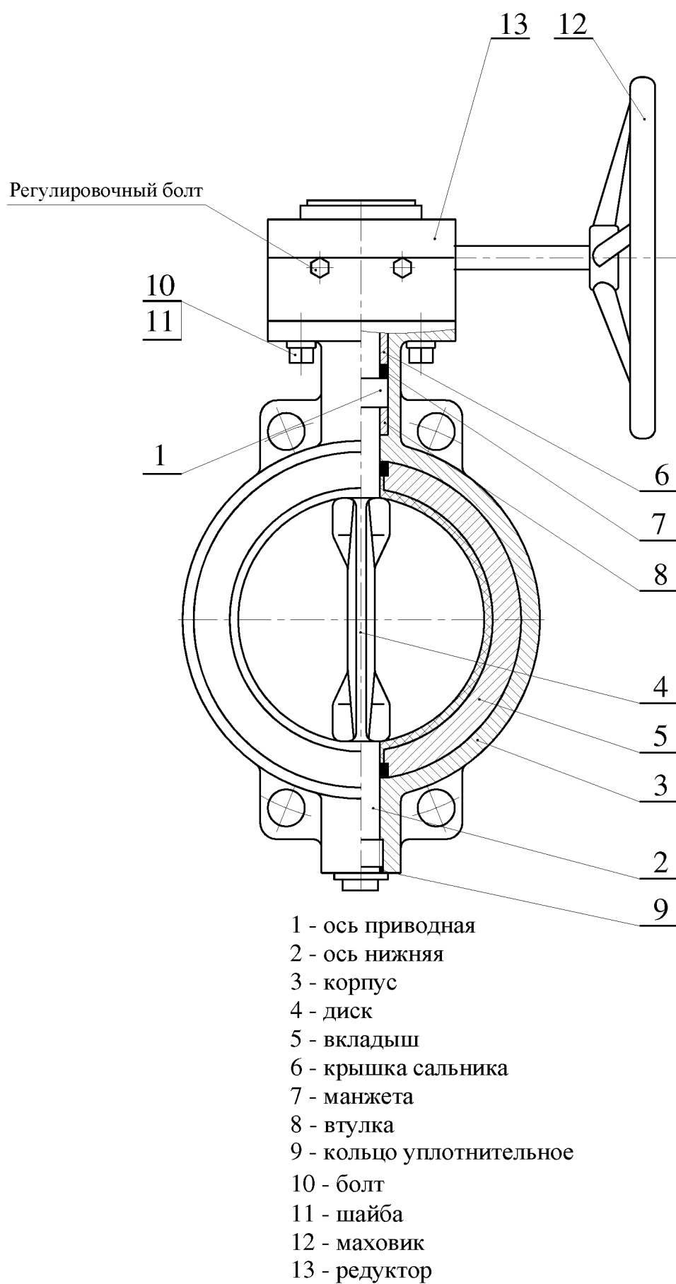
Рис. 4. Затвор с редуктором.
