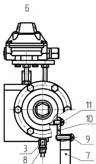
Рис. 7. Пневмогидропривод с БКВ «А-250» и пневмораспределителем.
