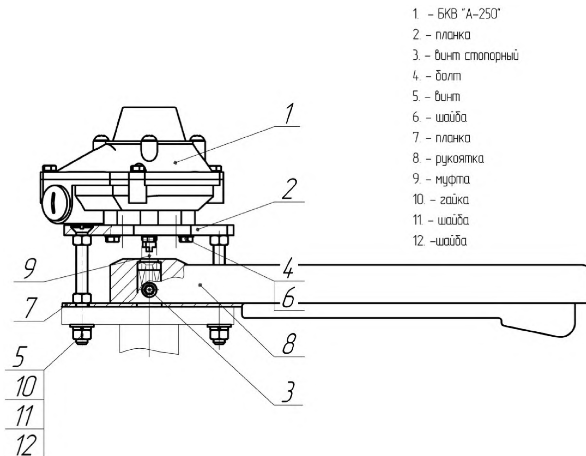
Рис.3. Установка БКВ «А-250» на рукоятку.
